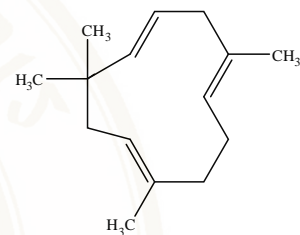
\alpha -humulene
