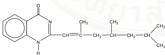
[2-(2', 4', 6'-trimethyl heptenyl)-4-quinazolone]
