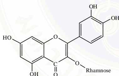
quercitrin (quercetin-3-O-rhamnoside)
