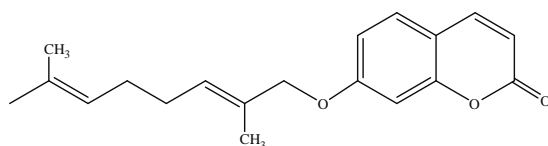
aurapten
