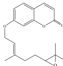
epoxyaurapten
