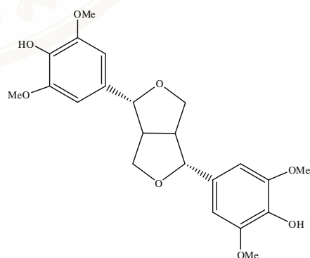
(+)-syringaresinol
