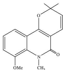
zanthobungeanine
